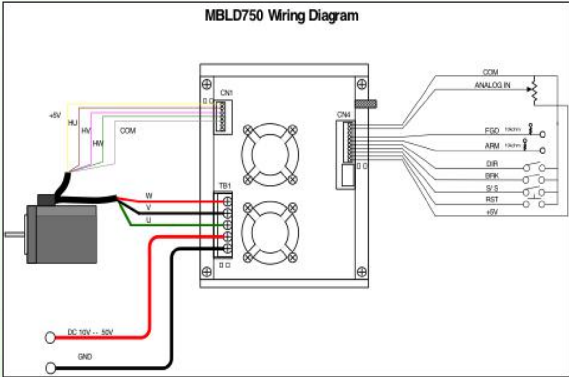
図3 MBLD750 モータ、ドライバー配線図
