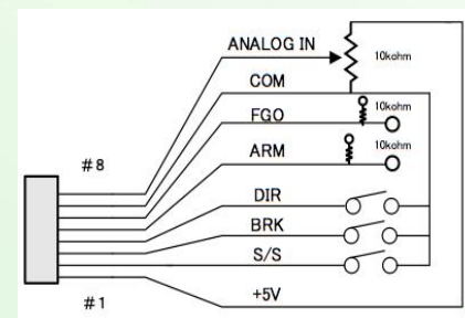
図2 CN5信号処理例
